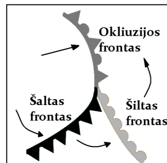
6.7 pav. Atmosferos frontų žymėjimas ir pagrindinės oro srautų judėjimo kryptys
