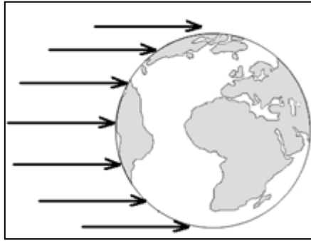
3.4 pav. Saulės spinduliuotės srautas konkrečiu laiko momentu (tik maža dalis Saulės spindulių krinta statmenai paviršiui)
