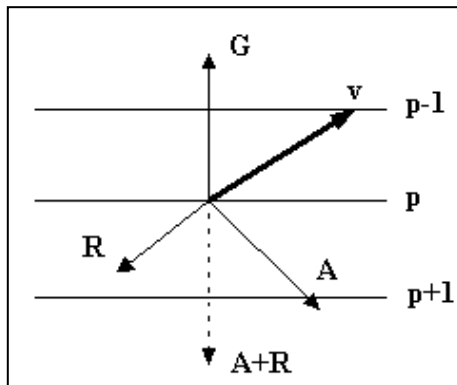
5.24 pav. Vėjas trinties sluoksnyje esant tolygiam ir tiesiaeigiam judėjimui: G – barinio gradiento jėga, A – Koriolio jėga, R – trinties jėga, v – vėjas
