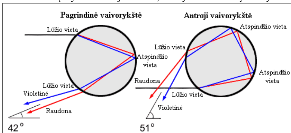
8.5 pav. Pagrindinės ir antrosios vaivorykštės formavimasis
