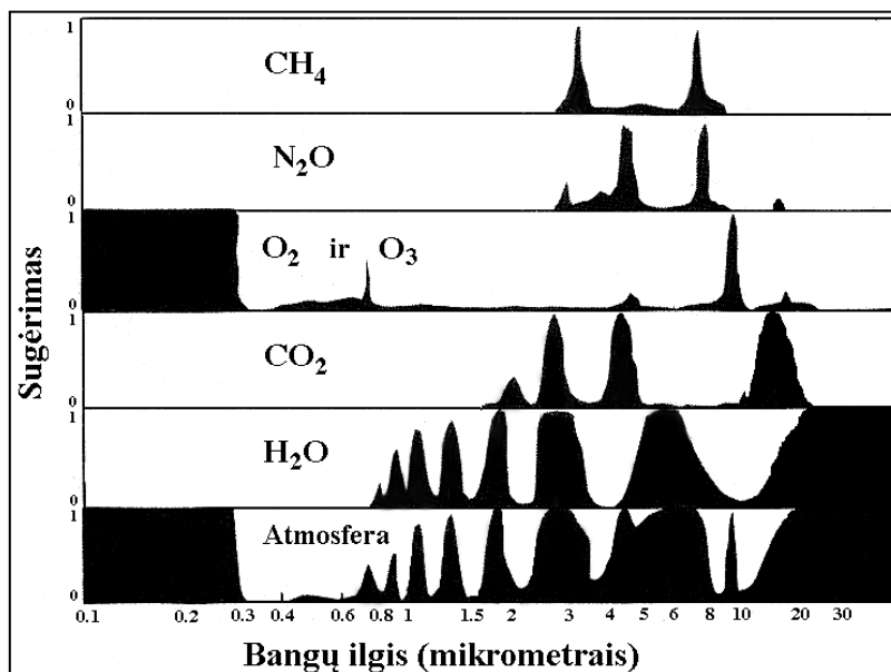
3.6 pav. Selektyvus įvairaus ilgio elektromagnetinių bangų sugėrimas atmosferoje. Pateiktos kai kurios daugiausia spinduliuotės sugeriančios atmosferos dujos (Nese, Grenči, 2001)
