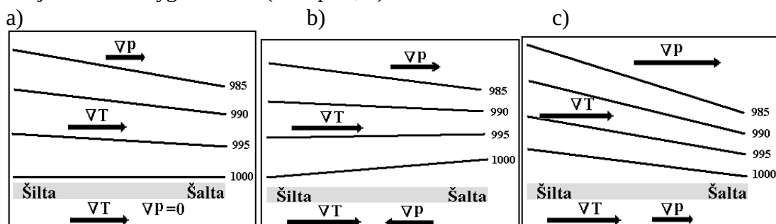
5.15 pav. Barinio gradiento krypties kaita didėjant aukščiui: a) barinis gradientas prie paviršiaus lygus 0, b) barinio gradiento kryptis prie paviršiaus yra priešinga temperatūros gradiento krypciai, c) barinio gradiento kryptis prie paviršiaus sutampa su temperatūros gradiento kryptimi
