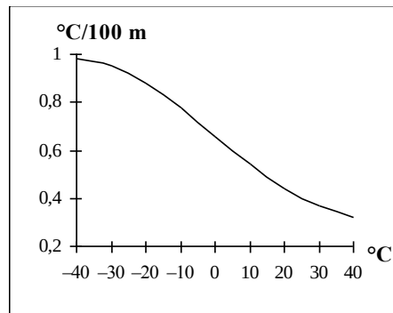
4.2 pav. Drėgnojo adiabatinio gradiento priklausomybė nuo vandens garų prisotinto kylančio oro tūrio temperatūros ( p = 1000\text{ hPa} )
