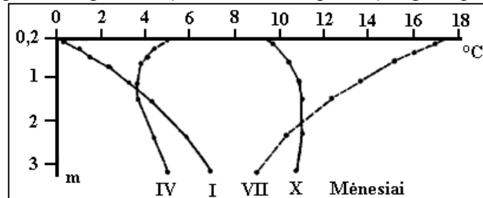
4.16 pav. Dirvos temperatūros (po augaline danga) kaita vertikaloje pagal Kauno agrometeorologijos stoties duomenis (Bukantis, 1994)
