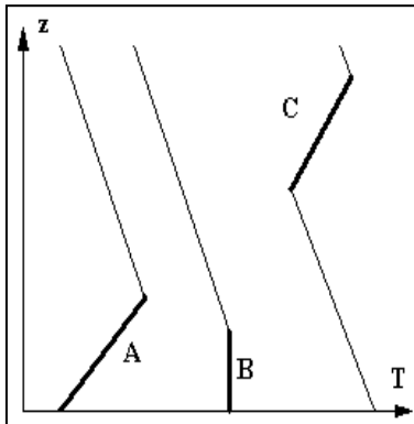
4.6 pav. Temperatūros vertikaliosios kaitos tipai: A – priežeminė inversija, B – priežeminė izotermija, C – pakilioji inversija
