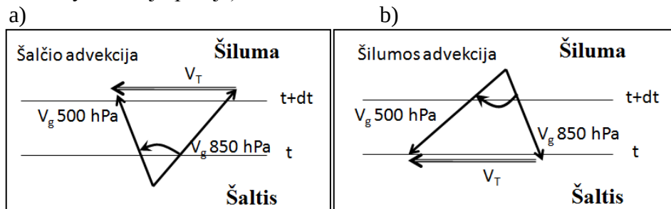
5.22 pav. Geostrofinis vėjas sukasi prieš laikrodžio rodyklę esant šaltio advekcijai (a) ir pagal laikrodžio rodyklę esant šilumos advekcijai (b); v_T – terminis vėjas
