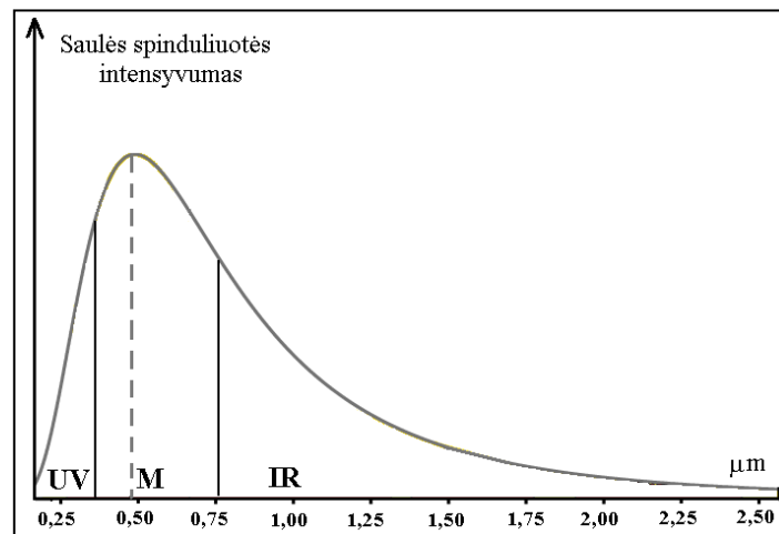
3.2 pav. Saulės spinduliuotės intensyvumo priklausomybė nuo bangos ilgio. UV – ultravioletinė spinduliuotė, M – matomoji, IR – infraraudonoji spinduliuotė. Intensyvumo maksimumas tenka 0,48\ \mu\text{m} ilgio bangai
