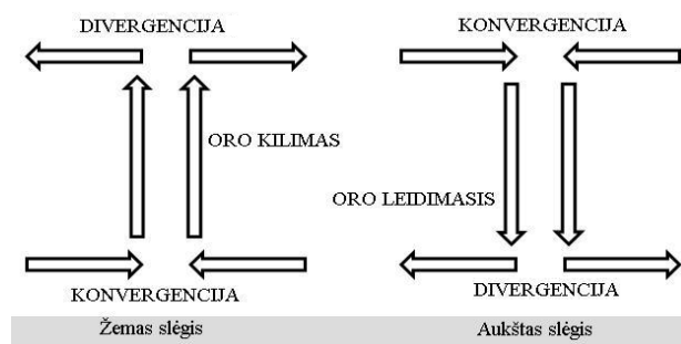
5.12 pav. Konvergencijos ir divergencijos ryšys su vertikaliaisiais oro srautais
