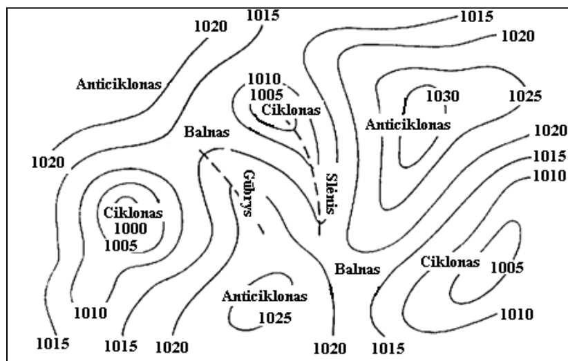
5.3 pav. Barinės sistemos (Gorodeckiy ir kt., 1991)
