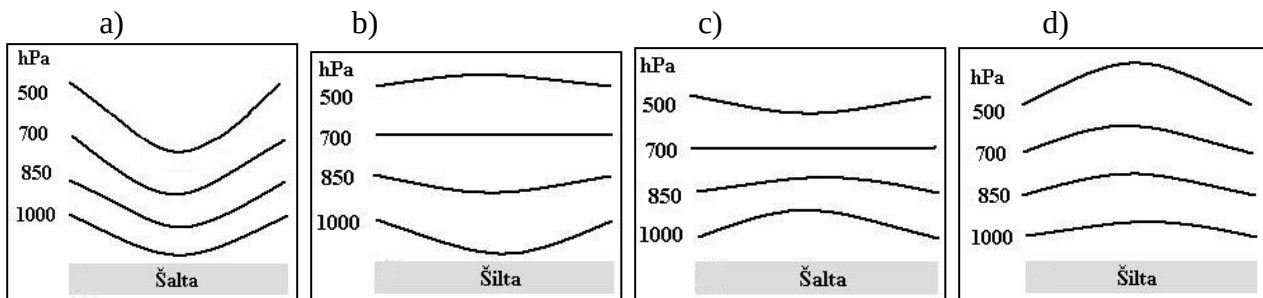
5.17 pav. Vertikalusis izobarinių paviršių pjūvis: a) aukštame (šaltame), b) žemame (šiltame) ciklone, c) žemame (šaltame), d) aukštame (šiltame) anticiklone
