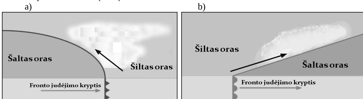
6.4 pav. Šaltojo (a) ir šiltuojo (b) atmosferos frontų schemas (Pidwirny, 2006)
