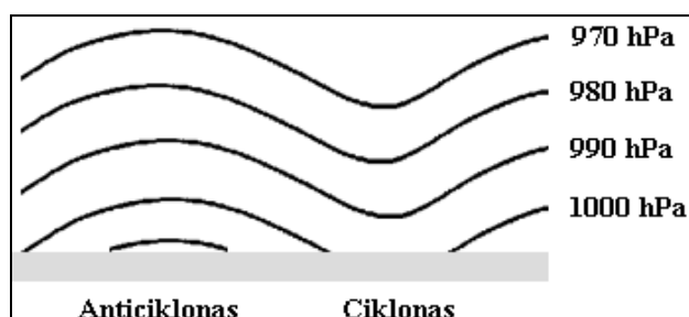
5.4 pav. Ciklono ir anticiklono vertikalūs izobarinių paviršių pjūvis
