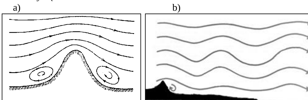
5.13 pav. Kalnų grandinės poveikis oro srauto judėjimui: a) priežeminių sukurių šlaituose susidarymas (Gorodeckiy ir kt., 1991), b) bangų pastoviai stratifikuotame ore formavimasis (Aviation Weather, 1975)
